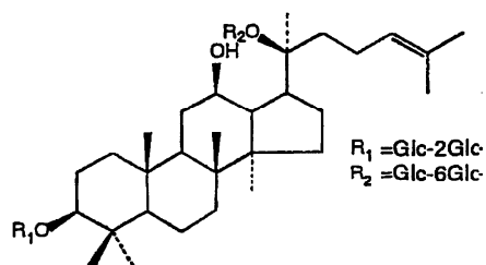
ギンセノシド Rb 1
